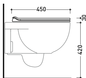
art. QK118 (fuori produzione / out of production) vista laterale / lateral view
