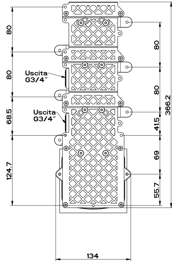
Vista dietro
